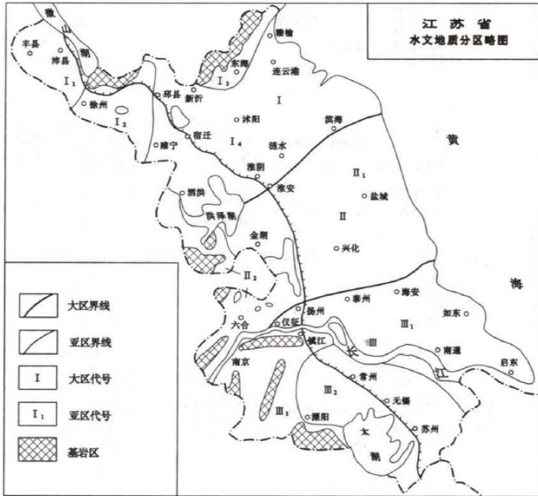
图 3.3-1 江苏省水文地质分区图
